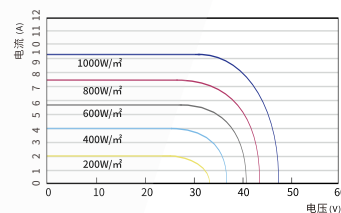
LNSF-335P/I-V
